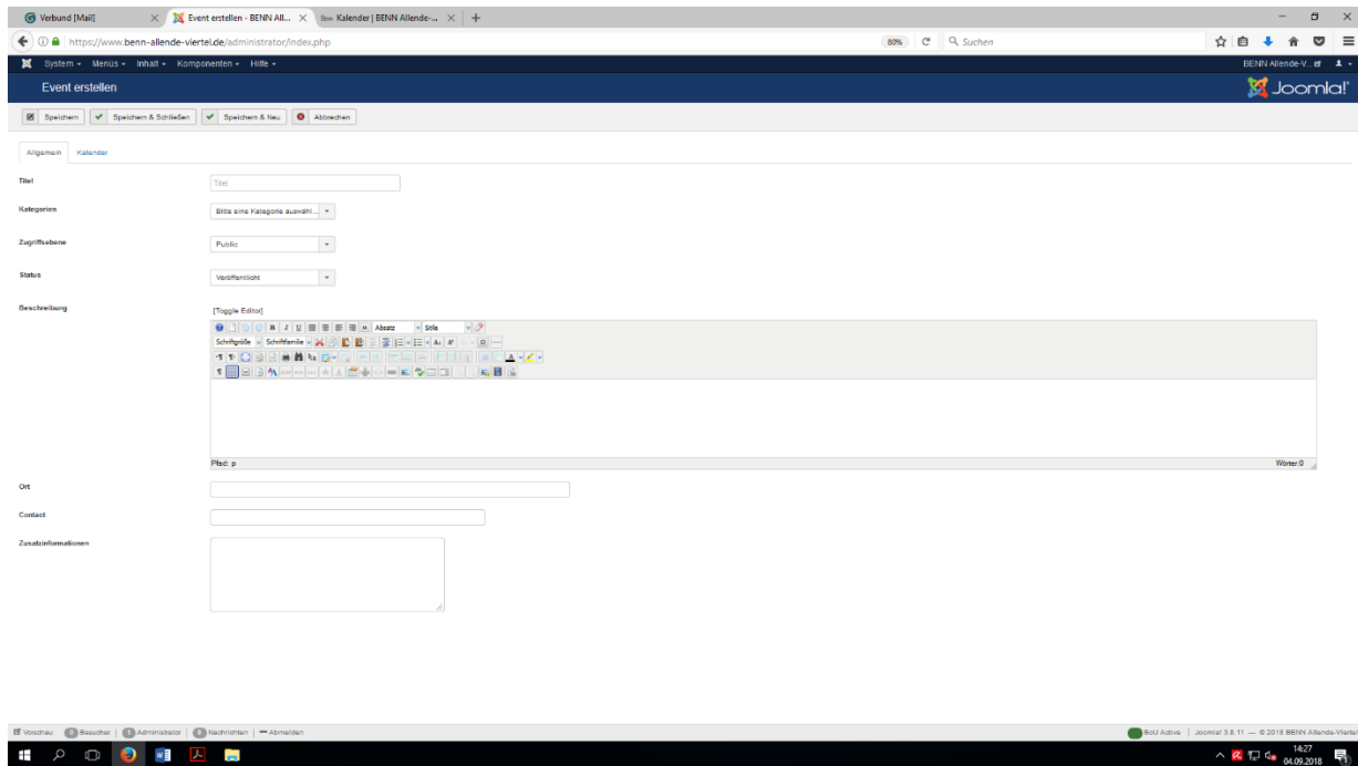
Abb. 04: Eingabemaske Veranstaltungskalender
